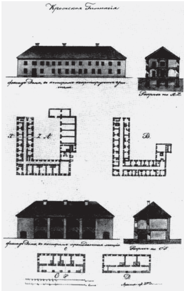
1827–1829 m. K. Podčiaišinskio iniciatyva sudaryti Kražių gimnazijos apmatavimo brėžiniai (CVIAP f. 733, ap. 96, b 20, l. 2)
