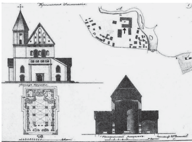
1827–1829 m. K. Podčiaišinskio iniciatyva sudaryti Kražių bažnyčios apmatavimo brėžiniai (CVIAP f. 733, ap. 96, b 20, l. 1)
