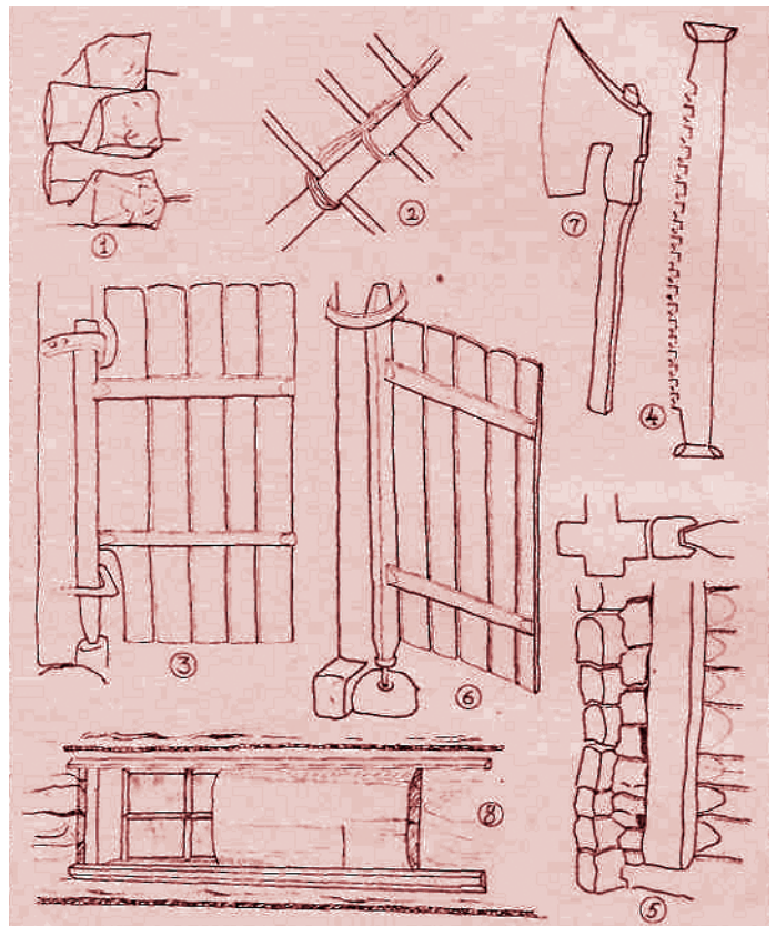
1 pav. 1. Šasparos „su kertėmis“. 2. Grebėstų pritvirtinimai. 3. Durys „ant bėgūnų“. 4. Skerspjūklis (Šiaulių „Aušros“ muziejaus eksponatas). 5. Rąstų sudūrimai. 6. Durų pastatymas ant akmens. 7. Skliutas (Šiaulių „Aušros“ muziejaus eksponatas). 8. Užstumiamas langas
